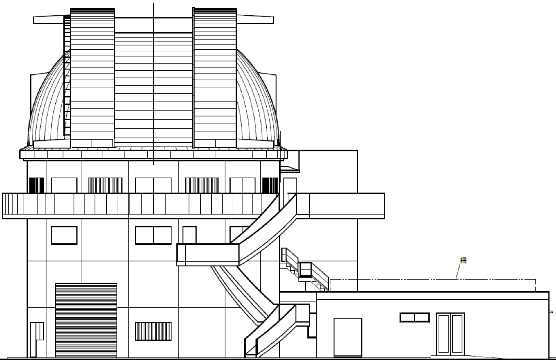
南面立面图
