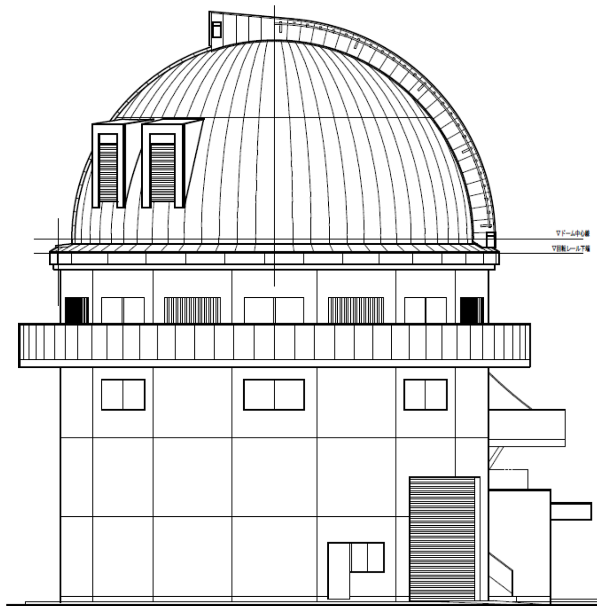
西面立面図
