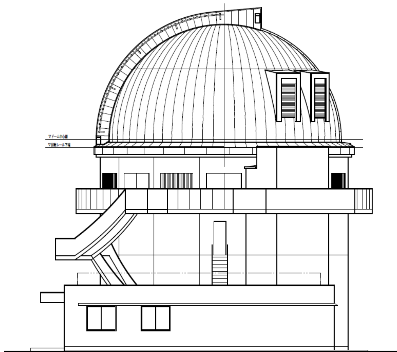
東面立面図
