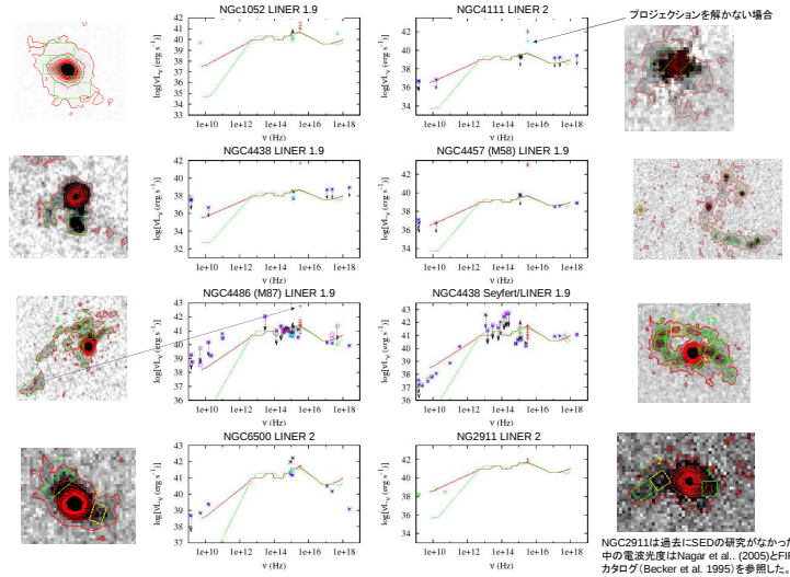
図6 AGN的な輝線比を示す輝線放射領域を持つLINERのSED。+が本研究で求めたUV光度。+とxはそれぞれMaoz (2007)とHo et al. (1999)のデータ。*は全てElacroux et al. (2010)のデータで、●は観測値。*とxはそれぞれCalzettiとSearsonの吸収補正を用いて吸収補正した値。赤線と緑線はradio loud quasarとradio quiet quasarのSED (Elvis et al. 1994)をスケールアップしたもの。各SEDの横にあるH \alpha イメージ上に、測定した輝線放射領域を示している。緑の領域の輝線比が0.8以上、黄色は0.8以下(ここに示している黄色い領域はどれも輝線比が0.7以上であった)。
