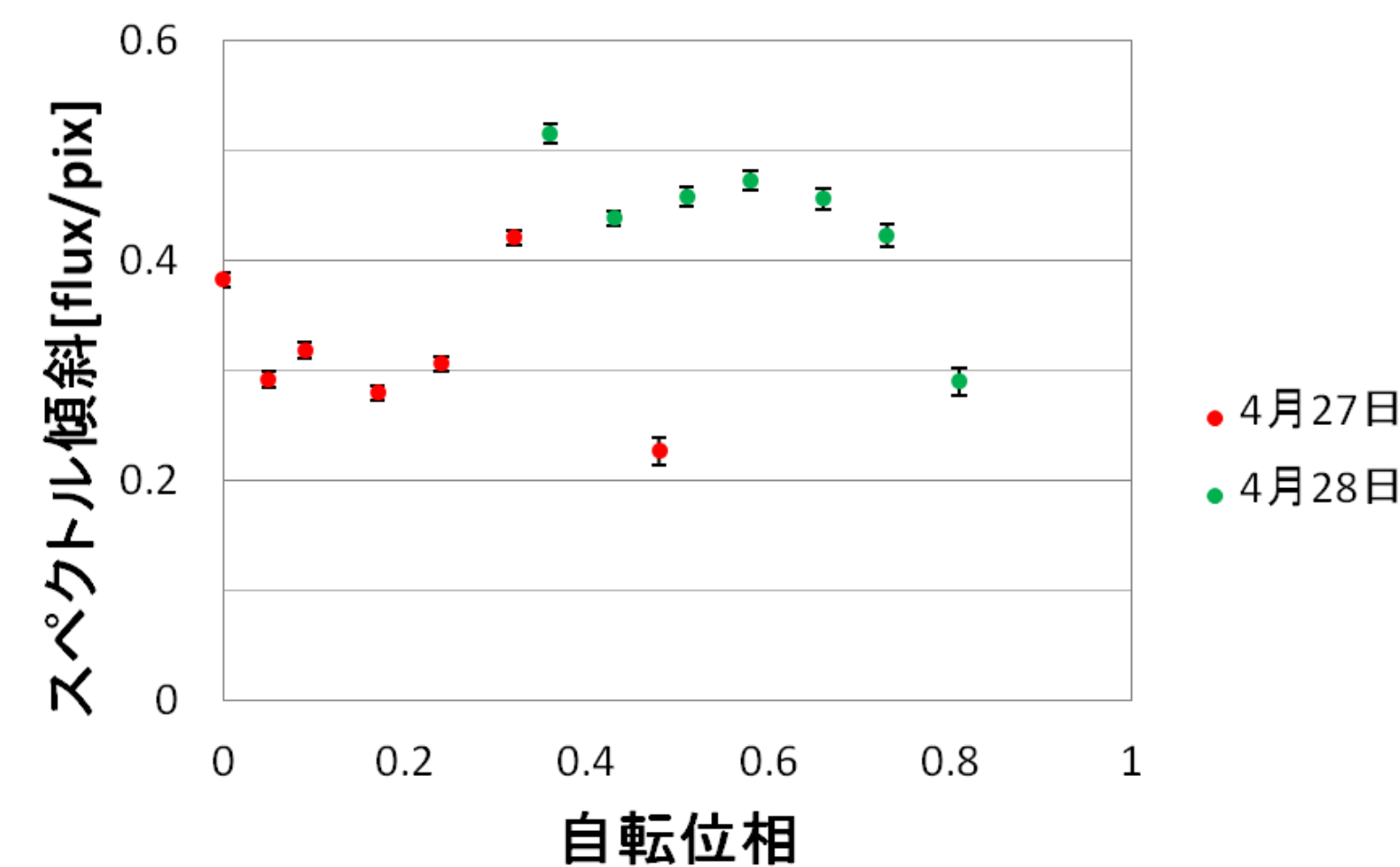
図3:位相と1.20μm-1.32μmの傾き
