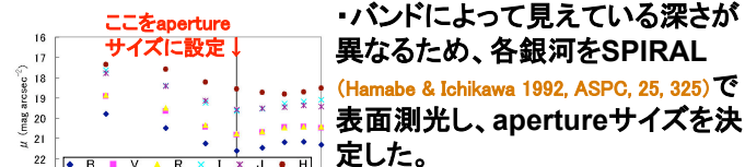
(図3: HCG55aの各バンドでの表面測光)
