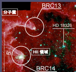
図1: Spitzerによる赤外画像(3.6 ~ 8.0 μm) (Koenig et al. 2008)
