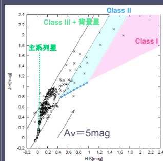
図3: BRC13の二色図
