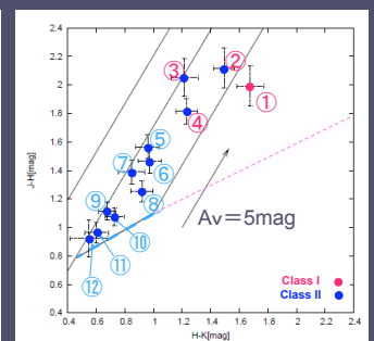
図3: BRC13の二色図
