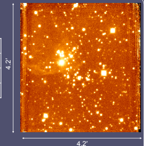
Fig.3: Hバンド重ね合わせ画像 30s×98frames = 積分時間: 2940s
