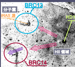
図2: DSS2 可視画像
