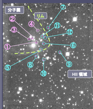
図4: YSO候補天体の空間分布
