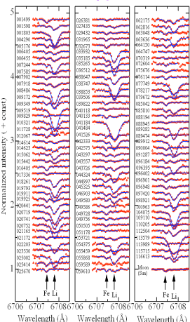
Li 6708線フィッティング グ(黒線:理論、色丸: 観測)
