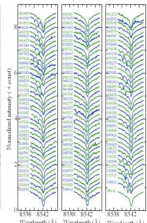
Call 8542線 コア付近のスペク トル
