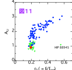
(5) 表面リチウム量と恒星活動(正の相関)
