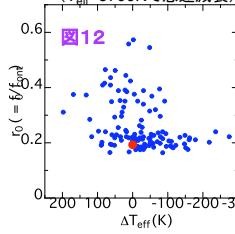
(6) 有効温度と恒星活動( T_{\text{eff}} < 5700 Kで急速減衰)
