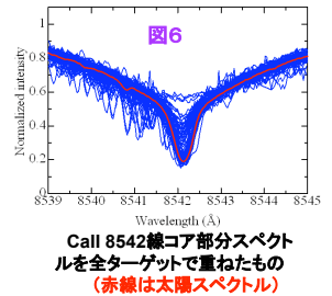
Call 8542線 コア付近のスペク トル
