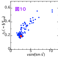
(4) 恒星活動と自転速度(正の相関)
