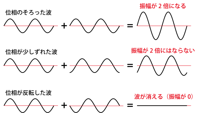
02 波の干渉。
