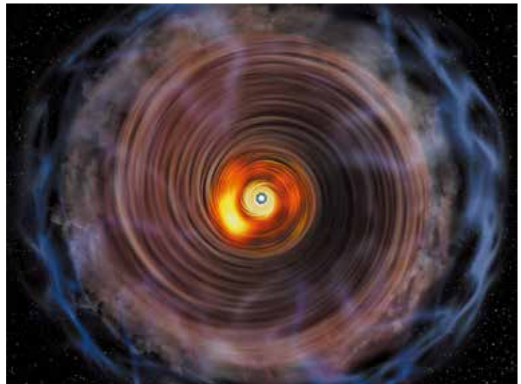
図01 アルマ望遠鏡での観測をもとに描いた巨大原始星 G353.273+0.641の想像図。中央にある原始星を取り巻く円盤を真上から見下ろすような位置関係にあり、円盤の構造をはっきり見分けることができる様子を表現しています。(Credit: 国立天文台)
