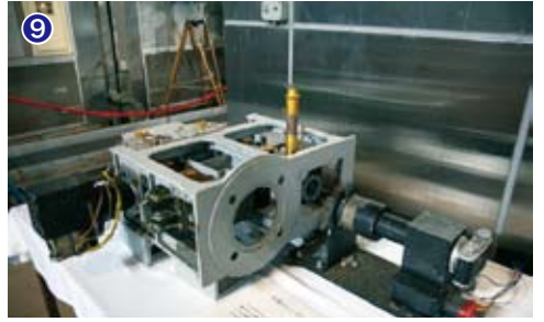
9 太陽カルシウム K 線分光器：サイテロスタットの太陽光からカルシウム K 線を取り出す分光器。
