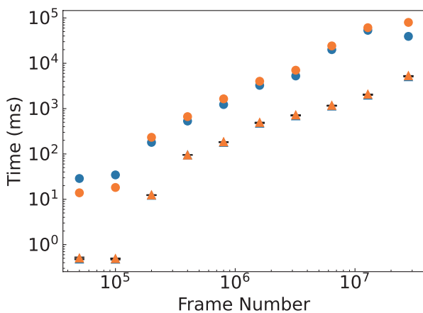
図3 ラフ検索のデータ総数と実行時間. 測定点の表示方法 (印の種類と色) は図2と同様である.
