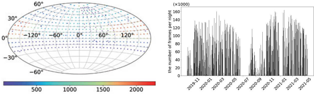
図1 左：実験用データのショットの中心座標の天球面上の分布．各点の半径1度以内にその中心座標が含まれるショットの数をカラーバーで示した色で表している．右：各観測日に取得されたスタック済みデータの数の分布．
