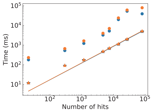
図6 ラフ検索のDISTINCT前の検索ヒット数と実行時間. 測定点の表示方法（印の種類と色）は図2と同様である. 対数プロットのため、検索ヒット数が0の実行時間は除いている. 青と橙の直線はキャッシュ有効時のテーブルの測定結果に対する回帰直線 ( y = 0.348x^{0.848} ) とビューの測定結果に対する回帰直線 ( y = 0.346x^{0.853} ) を表す.
