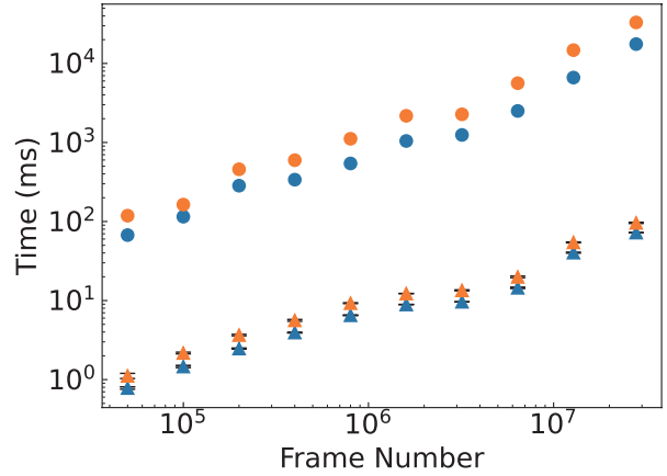
図2 ピンポイント検索のデータ総数と実行時間。青はテーブルを対象とした測定結果であり、橙はビューを対象とした測定結果である。それぞれ、丸はキャッシュが無効な場合、三角はキャッシュが有効な場合の測定結果である。キャッシュ有効時は4回の測定をおこないその平均を測定結果とし、その標準偏差を誤差棒で示した。
