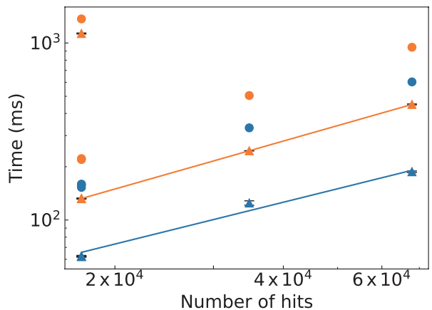
図7 カレンダー検索のDISTINCT前の検索ヒット数と実行時間. 測定点の表示方法（印の種類と色）は図2と同様である. 対数プロットのため、検索ヒット数が0の実行時間は除いている. 青と橙の直線はキャッシュ有効時のテーブルの測定結果に対する回帰直線 ( y = 0.031x^{0.784} ) とビューの測定結果に対する回帰直線 ( y = 0.020x^{0.900} ) を表す.
