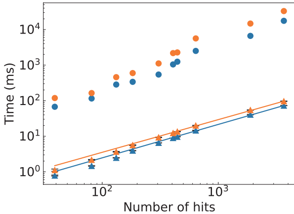
図5 ピンポイント検索の検索ヒット数と実行時間. 測定点の表示方法（印の種類と色）は図2と同様である. 青と橙の直線はキャッシュ有効時のテーブルの測定結果に対する回帰直線 ( y = 0.033x^{0.939} ) とビューの測定結果に対する回帰直線 ( y = 0.051x^{0.919} ) を表す.
