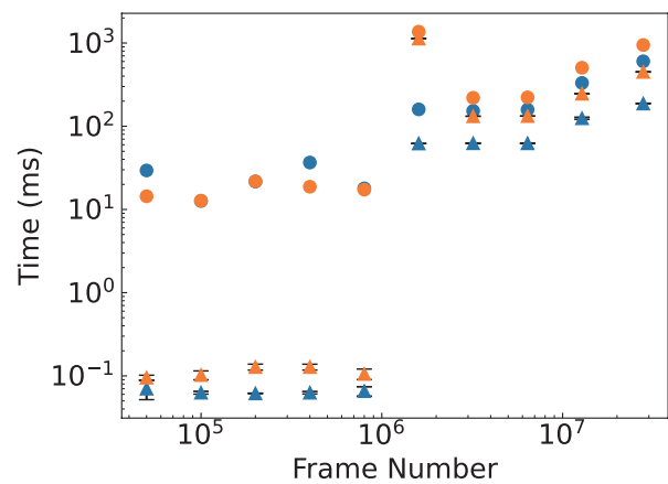
図4 カレンダー検索のデータ総数と実行時間. 測定点の表示方法 (印の種類と色) は図2と同様である.
