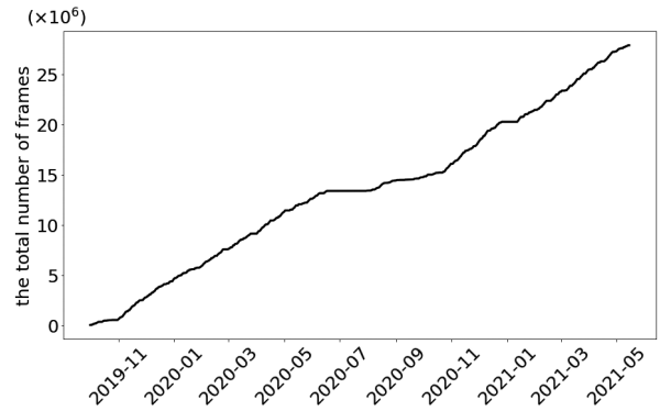
図8 本実験で使用したスタック済みデータのフレーム数の観測日に対する累積グラフ。一日平均4.7万フレームずつ増加している。
