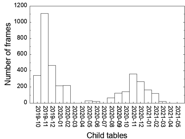
図9 date_obs列を分割キーとした分割テーブルに対するピンポイント検索 (SQL 4) の子テーブルあたりのヒット数。
