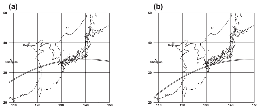
図4 紀元681年11月3日(天武10年9月17日)の月による火星の掩蔽. ×印は長安(Chang'an)と北京(Beijing). (a) \Delta T = 2000 秒, (b) \Delta T = 4000 秒. 曲線より下の地域では火星が月に隠れる.
