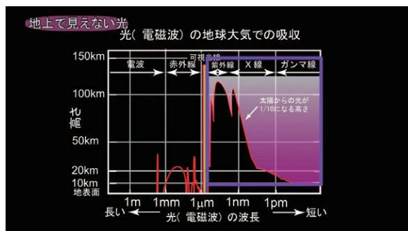
図13 地上では見えない光
