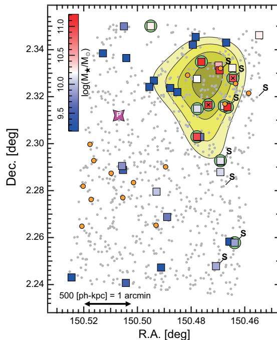
図1. 本研究で発見した赤方偏移2.16の原始銀河団 PHzG237領域における銀河の分布。すばる望遠鏡MOIRCSで同定したH \alpha 輝線銀河を四角印で表す（シンボルの色は銀河の星質量を表しており、赤いシンボルほど星質量が大きい）。緑色の丸印は中間赤外線検出されたH \alpha 輝線銀河、オレンジ色の丸印はハッセル宇宙望遠鏡で検出された遠赤外線ソース、プランク衛星のサブミリ波源の位置を「P」で、本研究で分光確認された原始銀河団のメンバー銀河を「S」で、X線源を「X」で表す。黄色のコントアは銀河団メンバー銀河の密度超過を表す。
