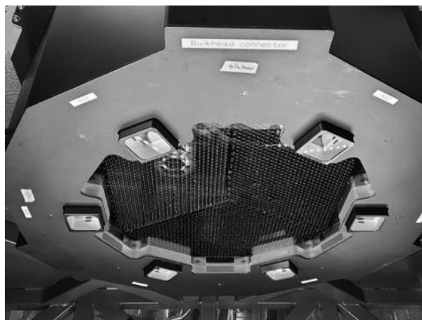
図2. PFI焦点面の様子。約2400本のファイバーとその配置モジュール、および6個の自動追尾カメラが見てとれる。
