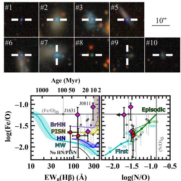
図1. (上) [2]で同定された9つの極金属欠乏銀河のHSC画像。(左下) Fe/OとH \beta 等価幅 (銀河年齢) との関係。データ点と曲線はそれぞれEMPRESSと化学進化モデルを表す。(右下) Fe/OとN/Oの関係。
