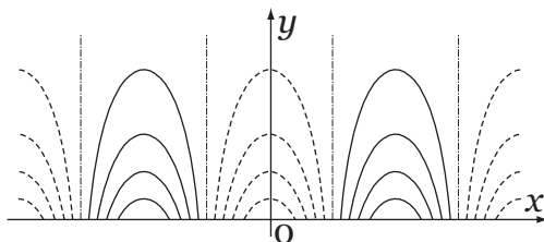
図8 Lamb wave ラム波 ( p' または \rho' )。
