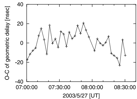
図 2. 群遅延解析から得られた幾何学的遅延時間とレンジ&ドップラ観測により推定された軌道から計算した幾何学的遅延時間の差。
