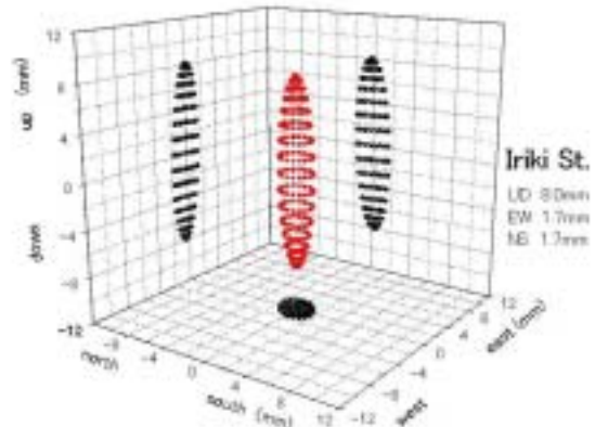
図 2. 水沢局を固定し、入来局の座標を求めた際の誤差楕円の例。水平位置の精度に対して上下位置は、時計や大気遅延とのパラメータ分離が悪いために精度が劣る。
