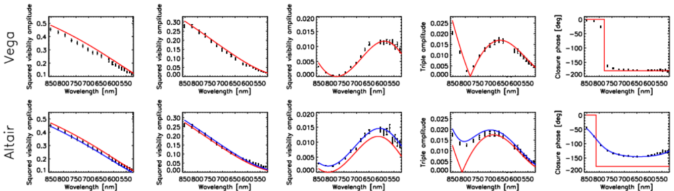
図 1. 2001 年 5 月 25 日の Vega (おりひめ; 上段) と Altair (ひこぼし; 下段) の観測データ。 V^2 は左から 29m, 37m, 64m 基線のもの。ベガのデータは、視直径 3.22mas の周縁減光モデル (赤線) によくあうが、アルタイル (3.32mas) では特に三重積の絶対値と位相があわない。周縁減光した楕円上に、輝点があると考える (青線) とよく説明できる。
