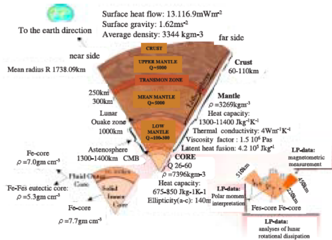
図 1. 種々の観測結果と理論的な検討から推定した月の内部構造。
