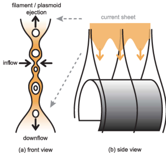
図1. 磁気リコネクションモデルの概念図。磁力線がつなぎ替り、上下両側にプラズマおよび磁力線が引き出される。
