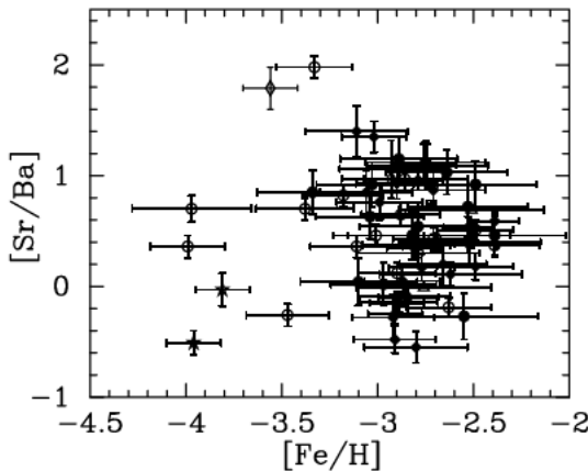
図 1. 過去の研究 (白丸) と今回の研究 (黒丸) によって得られた [\text{Sr}/\text{Ba}] を [\text{Fe}/\text{H}] の関数で示したもの。
