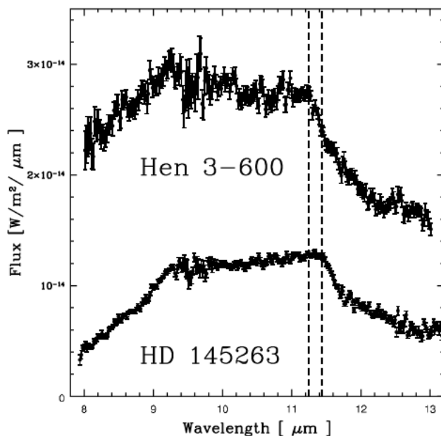
図 1. Vega 型星 HD145263 と T Tauri 型星 Hen3-600A の 8-13 \mu\text{m} スペクトル。スペクトルの長波長側の“肩”が Hen 3-600A は 11.24 \mu\text{m} であるのに対し、HD145263 は 11.44 \mu\text{m} と長波長側にシフトしている。この波長シフトは鉄を含むオリビンの出現の可能性があるのである (図 2 参照)。
