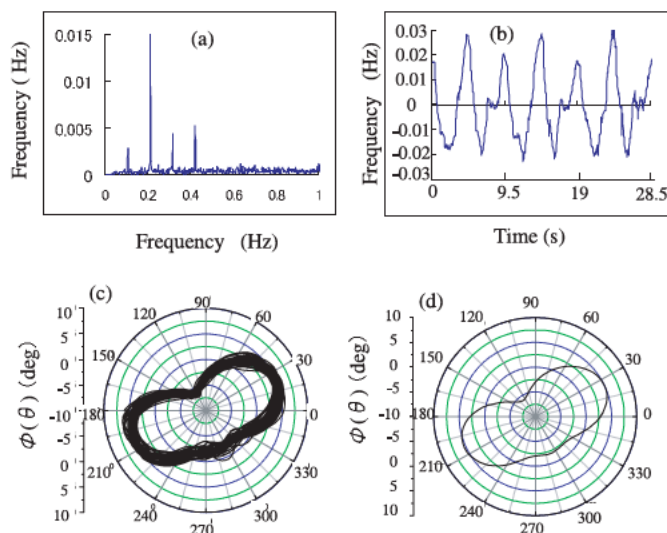
図 1. (a) ドップラー周波数のスペクトル, (b) f_{sp} とその整数倍の成分の時間変化, (c) (b) に示したデータを積分して計算した位相特性, (d) 平均処理後の位相特性
