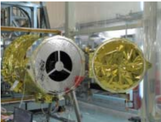
図 2. 可視光望遠鏡トップドア展開試験 (国立天文台・クリーンルーム)
