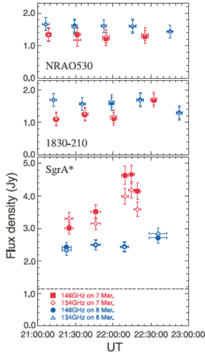
図 1. 2000 年 3 月 7-8 日の Sgr A* 及びキャリブレータ (NRAO 530, 1830-210) の 140 GHz 帯のライトカーブ [6]. 赤は 3 月 7 日を、青は 3 月 8 日を示す。3 月 7 日の Sgr A* のフラックス密度は、21:45 UT から 22:15 UT の間に 3.5 Jy から 4.7 Jy に増光している。点線は平静時の平均フラックス密度を示す。
