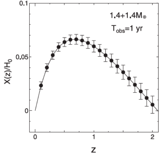
図2. 加速を表すパラメーター X(z) の振舞い。実線は \Lambda \text{CDM} ( H_0 = 75 \text{ km/sec/Mpc} , \Omega_M = 1 - \Omega_\Lambda = 0.3 ) の場合、中性子星連星の合体 1 年前から合体までのシグナルを ultimate DECIGO で検出する状況を考えている。縦棒のエラーバーはどの程度の観測誤差 ( 1\sigma ) で X(z) が決定出来るかを示す。
