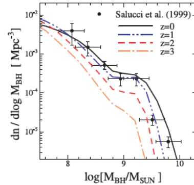
図 1. SMBH の質量関数の時間進化の予想 [2]. 誤差棒つきの黒点は z = 0 での SMBH の質量関数の観測結果 [3].
