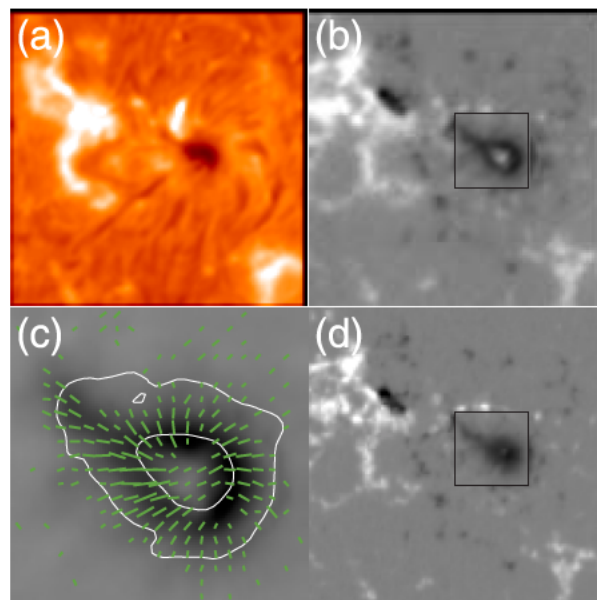
図 2. 2004 年 4 月 22 日に観測された NOAA 0596 の画像。(a-c) それぞれフレア望遠鏡による H \alpha 像、視線方向磁場を示す Stokes V/I 画像、直線偏光成分を加えた黒点部分の拡大像。(d) SOHO 衛星の MDI による光球磁場。(b)(d) 中の四角は、磁場が強いいためレベルを変えて表示した部分を示している。
