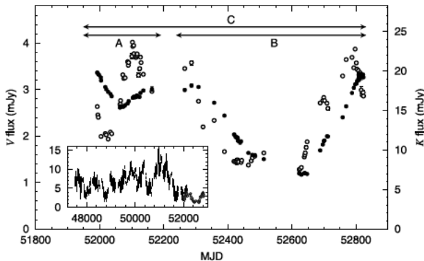
図 1. 2001 年 3 月～2003 年 7 月に観測された、NGC 5548 中心核の V バンド (○印) と K バンド (●印) の光度曲線。V バンドと K バンドの間の変動の時間差は、図中の A, B, C, それぞれの区間のデータについて計算した。小枠は、国際 AGN モニター協力組織が 13 年間観測した NGC 5548 の波長 5100 Å 連続波光度曲線データ (縦線) に、我々の V バンド光度曲線データ (○印) を重ねて表示したもの。
