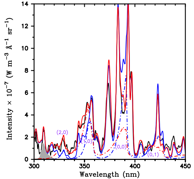
図2. 観測スペクトル(黒線)と、原子(温度4500 K)と分子( \text{N}_2^+(1-) : 赤線; 温度10000 K, 青線; 温度4400 K)を考慮した理論スペクトルとの比較。点線は、それぞれの温度における \text{N}_2^+(1-) の理論スペクトル。波長310 nm付近の灰色部は、OH A-Xバンドスペクトルである。OHの起源については、今後更なる確認が必要である。
