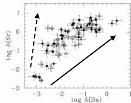
図 2. [\text{Fe}/\text{H}] \leq -2.5 の天体での \text{Sr} と \text{Ba} 組成の相関。実線矢印は \text{Sr} と \text{Ba} の増加を示す (main r -process)、破線矢印は \text{Sr} の増加を示す (weak r -process)。
