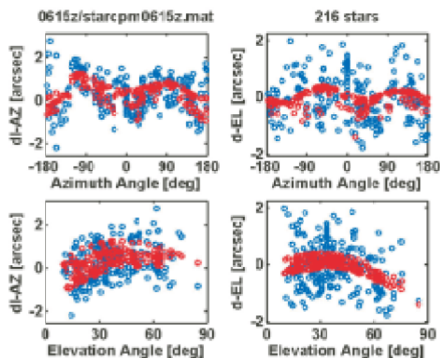
図 1. 光学望遠鏡を用いた全天絶対指向精度の測定。青丸が測定値 (Az 誤差は 0.85 秒角 rms, El 誤差は 0.80 秒角 rms, 絶対指向誤差は 1.17 秒角 rms), 赤丸がポインティング器差モデルフィット。
