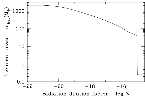
図1. 典型的な分裂質量と遠紫外線強度との関係。紫外線は10万度の黒体放射とし、その強度を希釈因子 W を用いてあらわしている。
