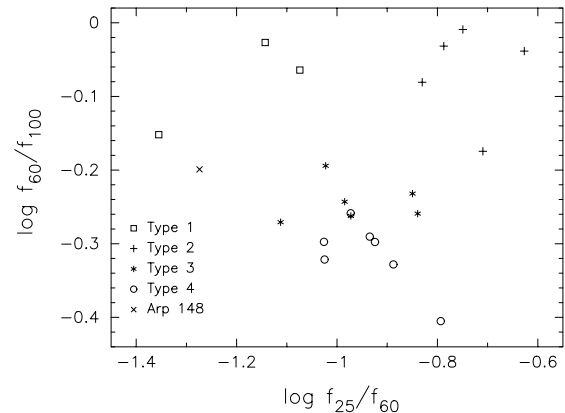
図3. 25, 60, 100 \mu\text{m} のフラックス比. タイプによって全く違う値を示している. このように、星形成領域の分布の仕方が遠く値を示している。
