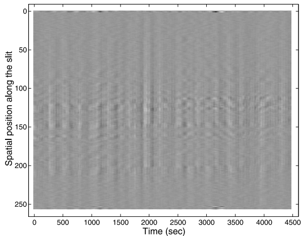
図1. 乗鞍コロナ観測所の分光観測による、コロナ緑色輝線の強度変動。縦軸はスリット方向の位置、横軸は時間である。右の図は、ゆっくりに変動する成分を差し引き、高周波成分を強調したもので、波動の伝搬の様子が見て取れる。
