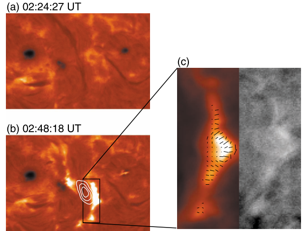
図2. 2002年10月14日のフレアのH \alpha 画像と偏光・速度場の観測結果。(a) フレア前のフィラメントを示す画像。(b) フィラメント消失後起こったtwo-ribbon フレア。コンタはRHESSIで観測された硬X線ソースを示す。(c) フレアリボンのうち(b)の四角の領域における偏光(左側)と速度場(右側)。短い棒が直線偏光の方向と偏光度を示しており、またDopplergramでフレアリボン中に白く表示されている部分はred shiftに対応している。
